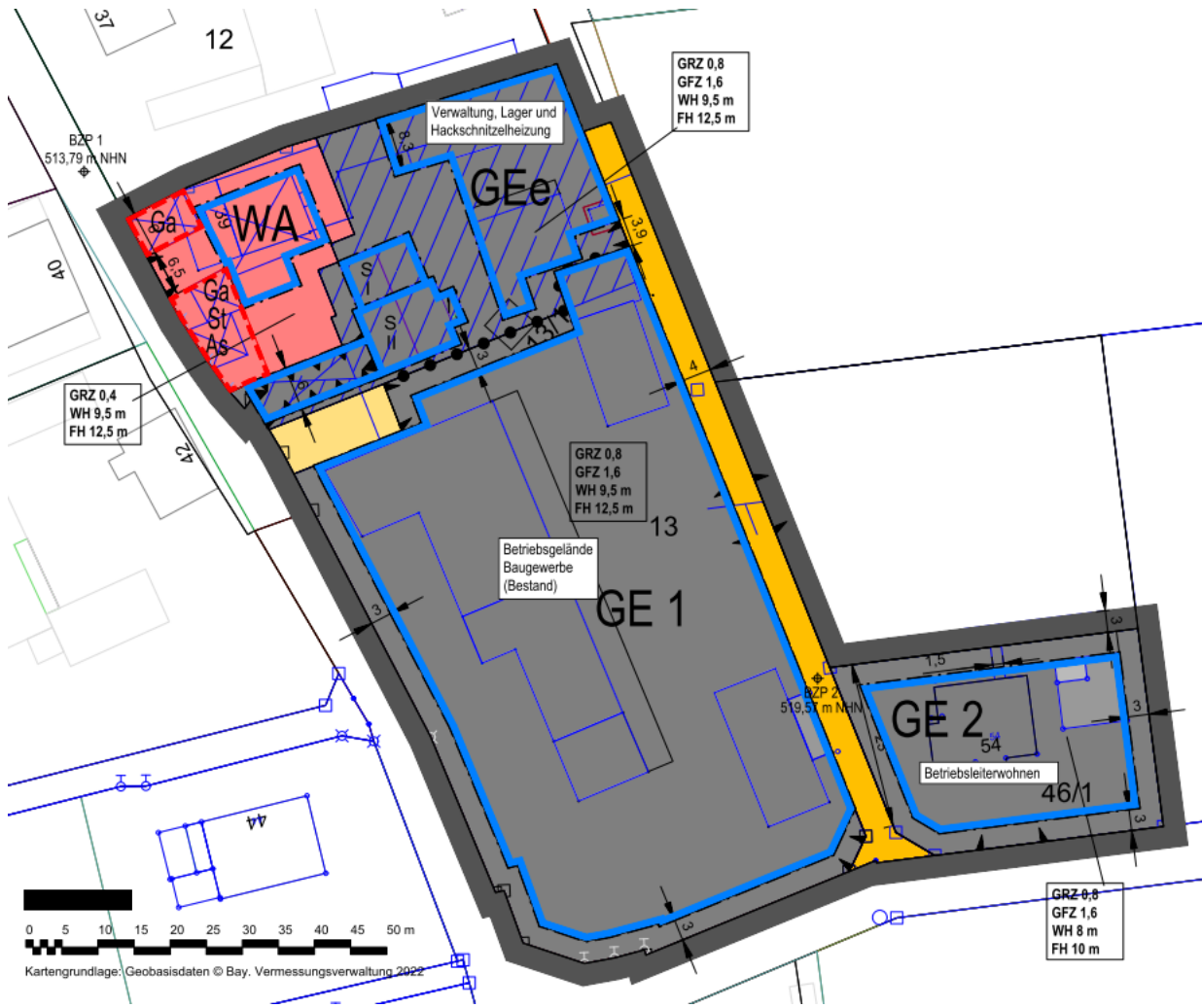
Planskizze mit Darstellung der für den B-Plan vorgesehenen Flächenaufteilung
