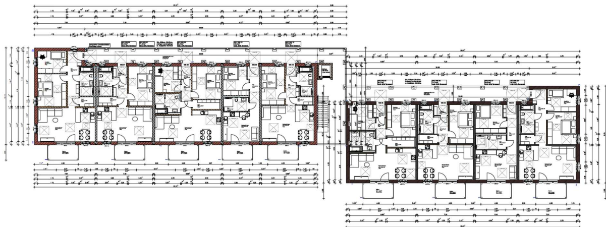
Grundriss Regelgeschoss
